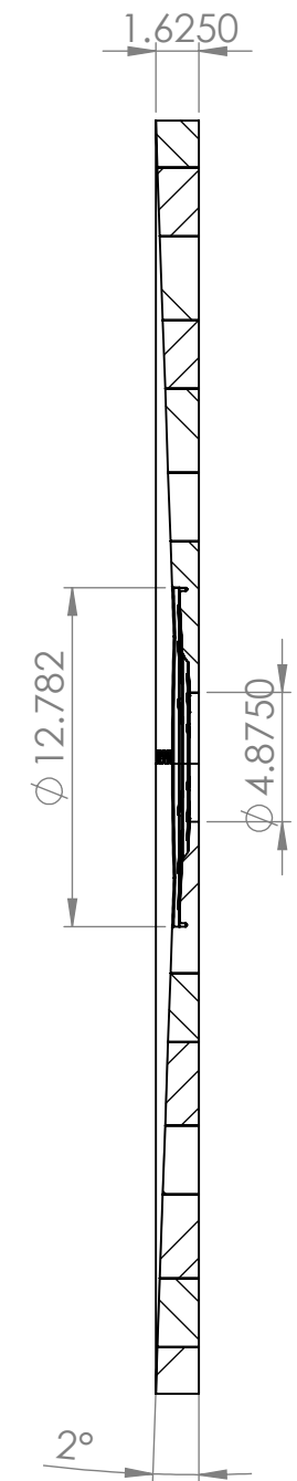
SECTION A-A
